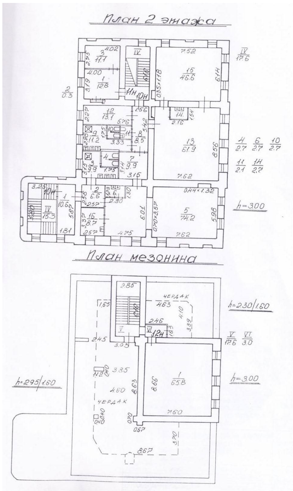
33. Современные планы второго этажа и мезонина.
