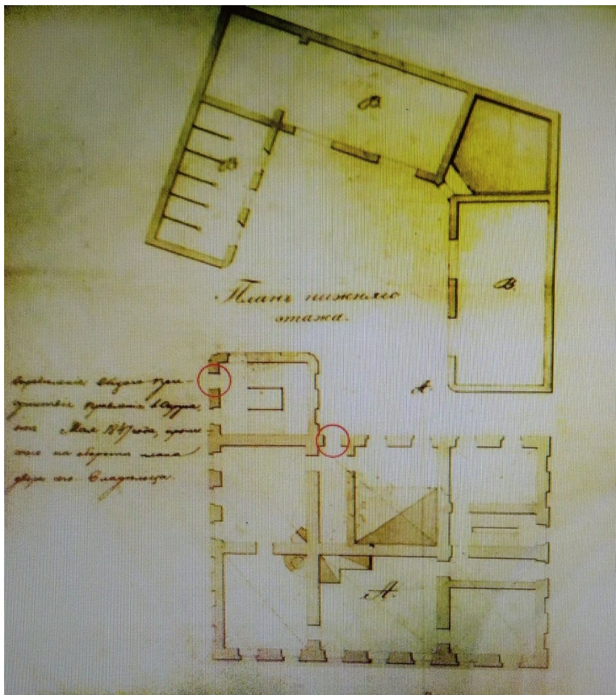
10. План нижнего (цокольного) этажа дома Губернского секретаря Друри. 1847 г.
