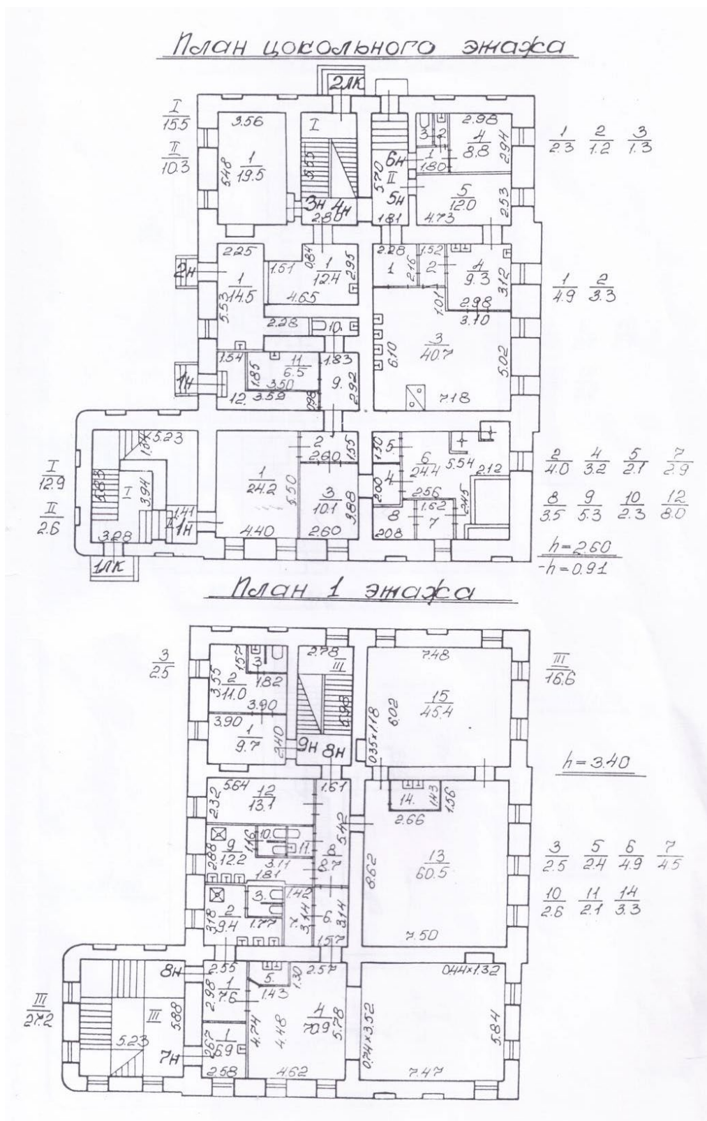
32. Современные планы подвального (цокольного) и первого этажей.
